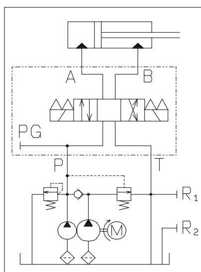
図1 油圧回路図
